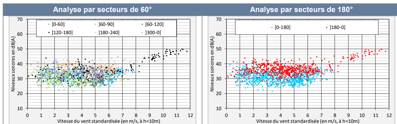
Planche 3 - Echantillons de bruit résiduel au point PF1 (Nuisement-sur-Coole), de nuit
